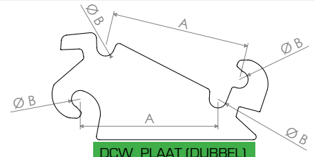
DCW_PLAAT (DUBBEL)
